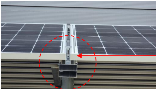
모듈 일체형 지붕 구조 프레임
