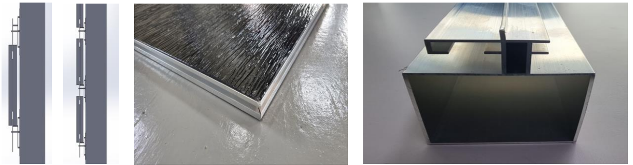
[샷시타입 모듈프레임 및 알루미늄 고정스터드]
