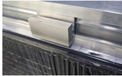
[Z-Bar 모듈프레임 및 Clip 고정스터드 알루미늄 프레임]
