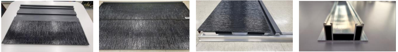
[강판 절곡 구조 및 PV 모듈과 일체형으로 접합, 알루미늄 고정스터드]
