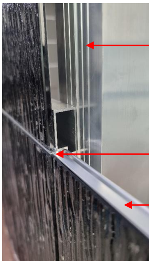
[스냅식 모듈프레임 및 오픈조인트 알루미늄 고정스테드]
